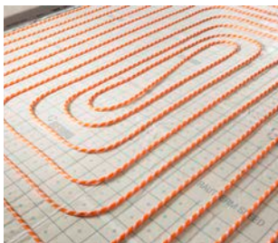
Obr. 21 Pokládací deska RAUTHERM SPEED s tepelnou a kročejovou izolací
