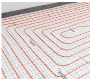
7. Hotová pokládka, proveďte tlakovou zkoušku
