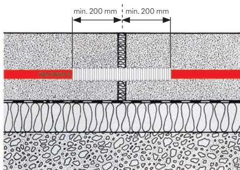
Obr. 172 Ochranná trubka při průchodu dilatační spárou
