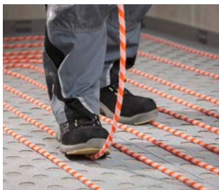
9. Pokládka trubky RAUTHERM SPEED K 10
