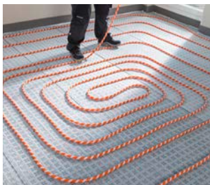
6a. Pokládka trubek na rohož
