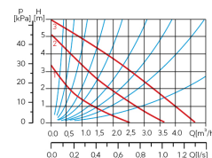
W0204 Oběhová čerpadla FERRO pro pitnou vodu
