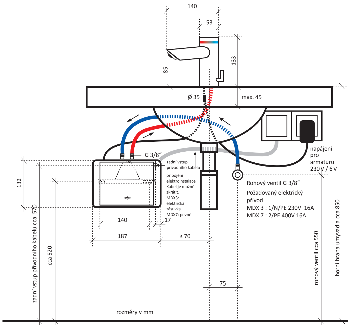
Příklad instalace s tlakovou armaturou
