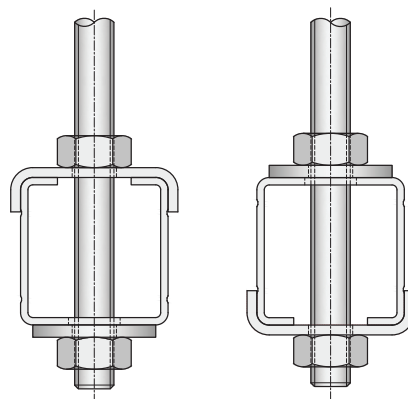
Obrázek 3: Použijte Walraven RapidRail® U-podložku na otevřené straně lišty
